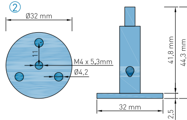
SA-001-002 Seilabhängungsset mit Montageplatte zur punktuellen Abhängung von PET Platten mit 2000x1,5mm Stahlseil Cable suspension set with mounting plate for selective suspension of PET panels with 2000x1.5mm steel cable
