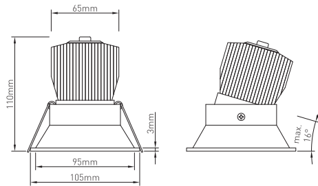
Deckenausschnitt / Ceiling Cutout: Ø 94 - 100mm Einbautiefe / Mounting Depth: 110mm
